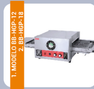
1. MODELO BB-HGP-12 2. BB-HGP-18 HORNO DE BANDAS A GAS CON ENTRADA DE 35 Y 50 CMS. 1. MEDIDAS: 1100 X 570 X 360 MM. 2. MEDIDAS: 1560 X 750 X 360 MM.
