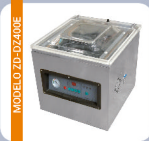
MODELO ZD-DZ400E EMPACADORA AL VACÍO MEDIDAS: 540 X 490 X 560 MM.
